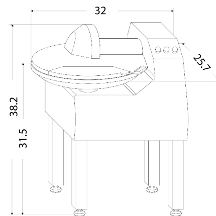
Dimensions TITANE 20
