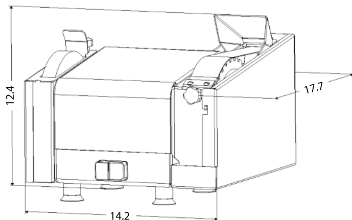
Dimensions RENOV 200
