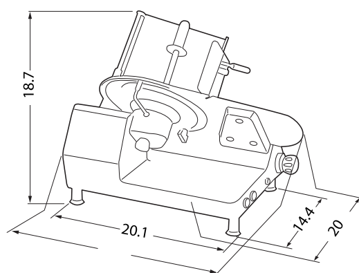
Dimensions GRAVINOX 300
