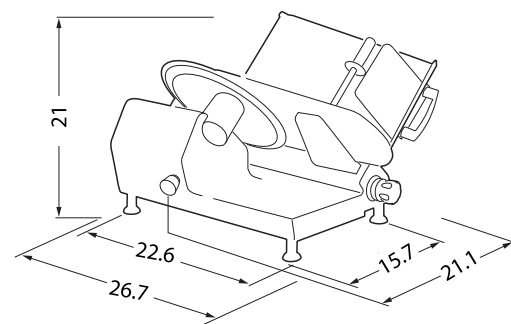
Dimensions GRAVINOX 350
